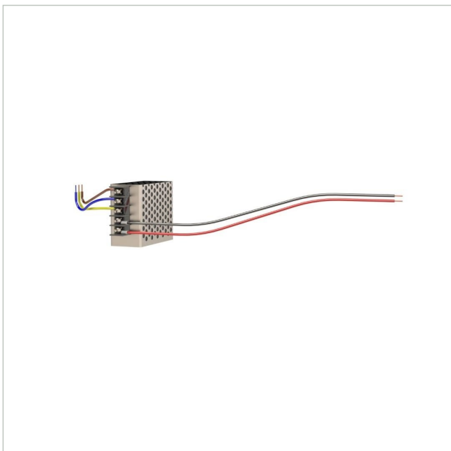
Netzteil 230/12VDC 1,3A für CSX814
